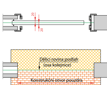
Dveře posuvné do pouzdra (do stěny)
