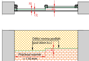
Dveře posuvné s bočním světlíkem – rámová konstrukce
